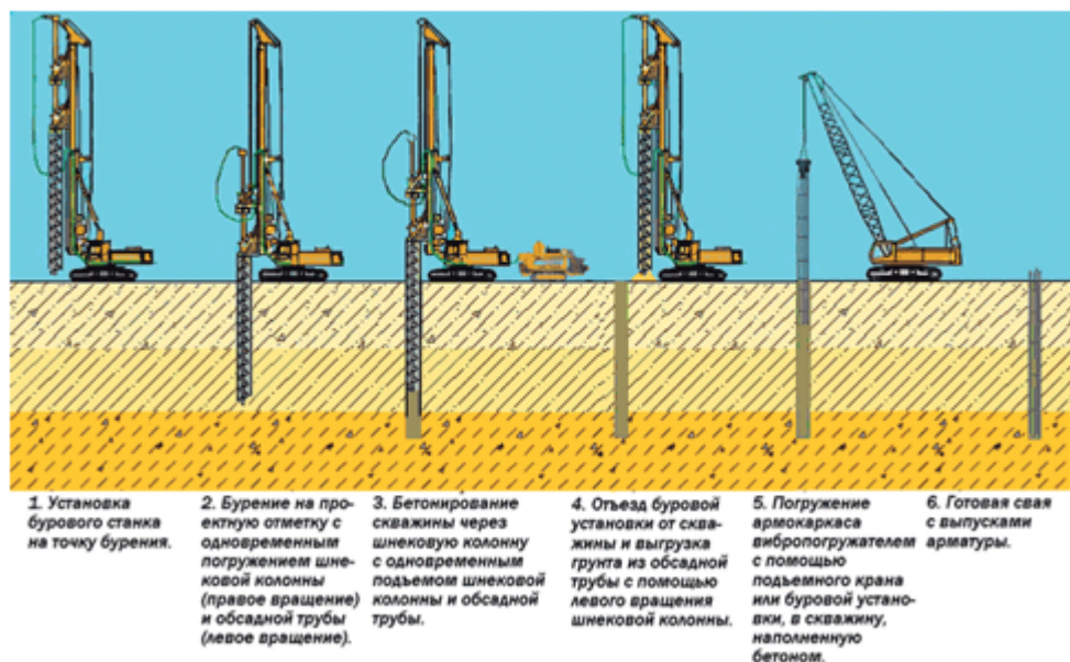
Рис. 11. Технологическая карта устройства буронабивных свай методом Double Rotary.
