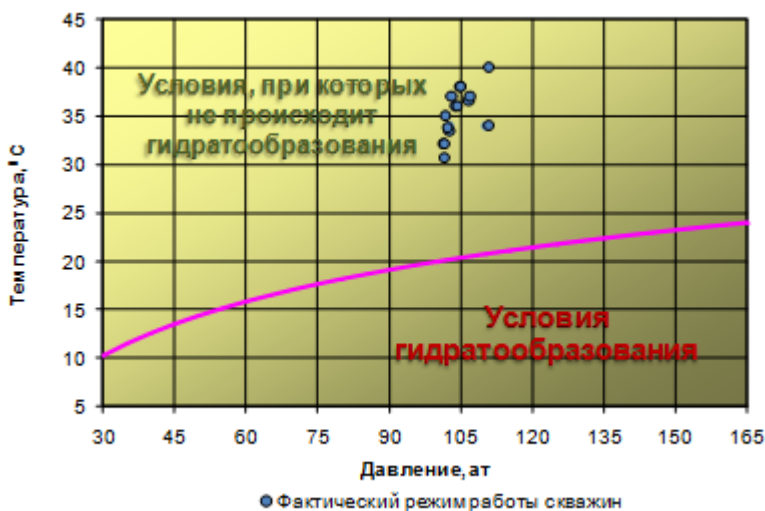
Рисунок 2 - Кривая гидратообразования
