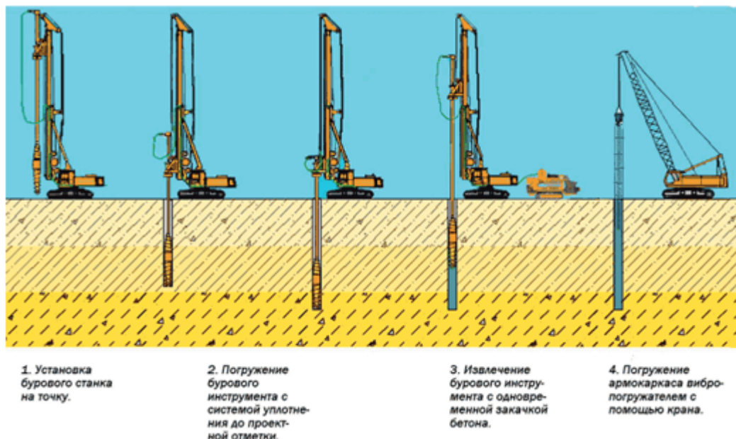
Рис. 12. Технологическая карта устройства набивных свай уплотнения DDS.
