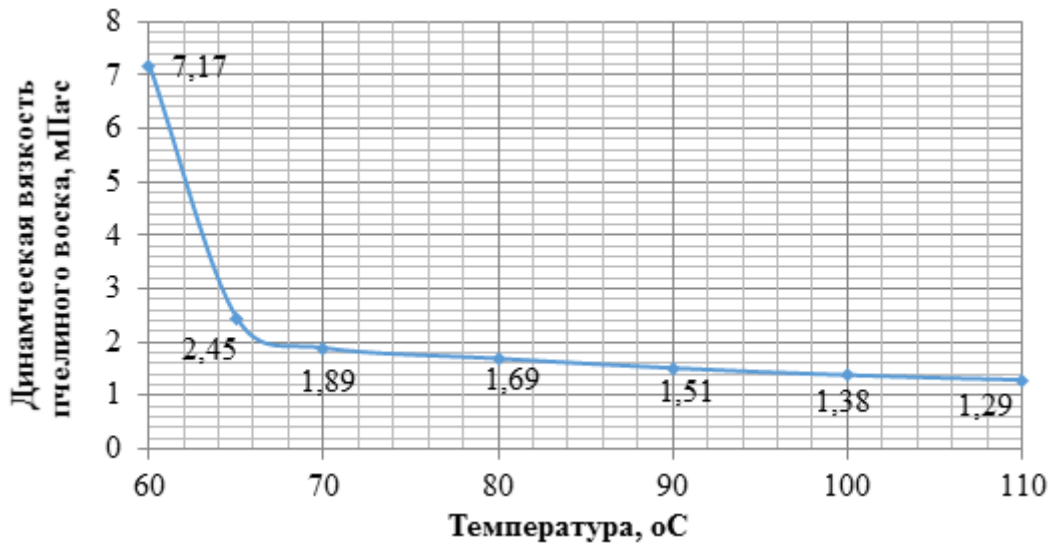
Рисунок 3 – Зависимость динамической вязкости воска от температуры нагрева
