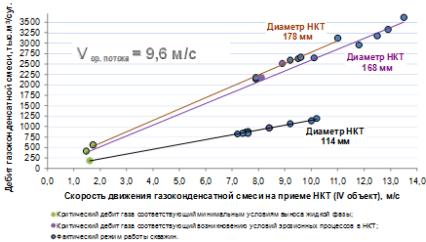
Рисунок 1 - Распределение скорости газоконденсатного потока на приеме НКТ в зависимости от производительности скважин
