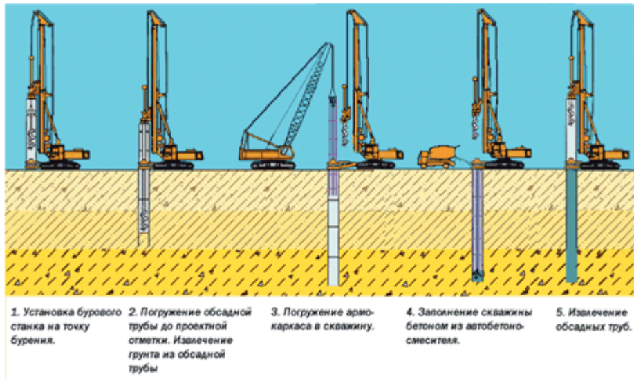
Рис. 2. Технологическая карта устройства свай под защитой обсадной трубы.
