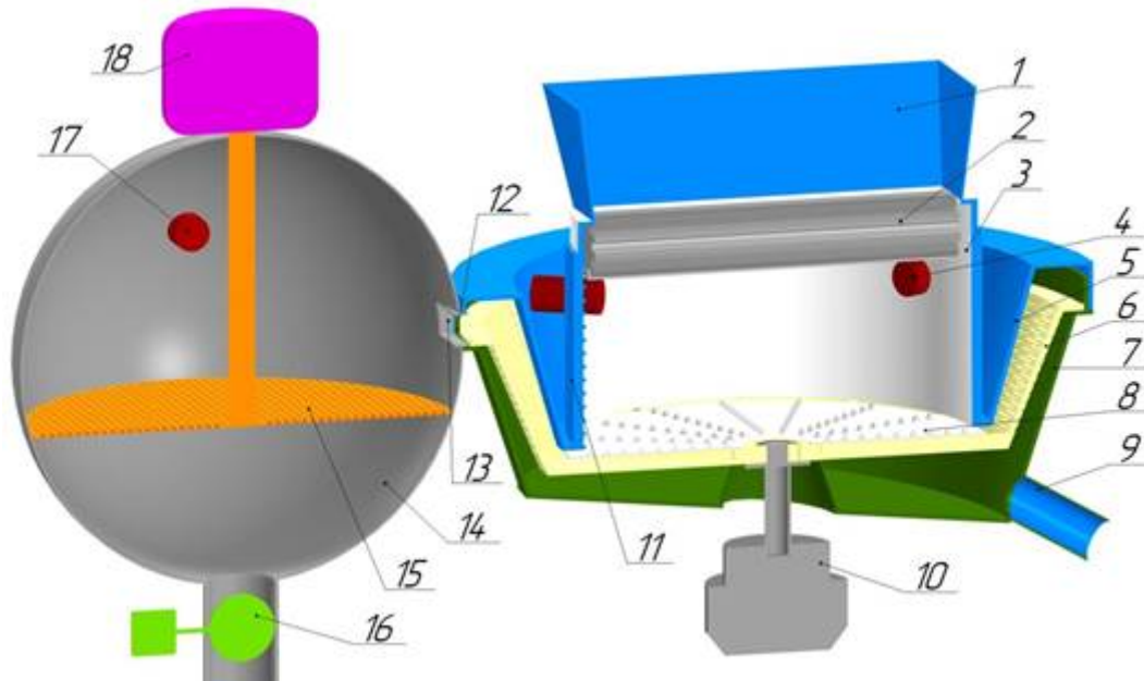
Рисунок 5 – СВЧ-установка для термообработки пчелиного воска:
