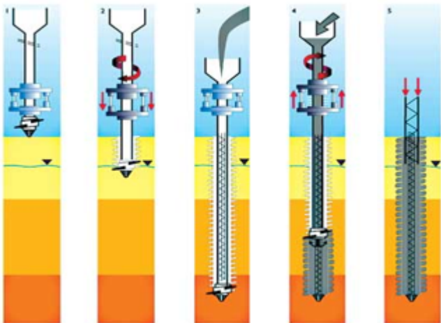
Рис. 14. Технология устройства свай Атлас.
