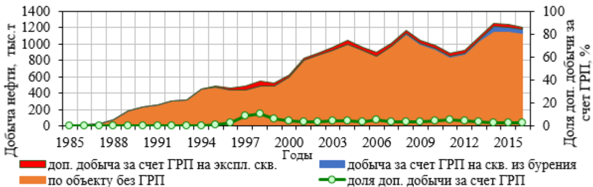
Рисунок 1 – Динамика добычи нефти по годам. Объект ЮВ 1 .
