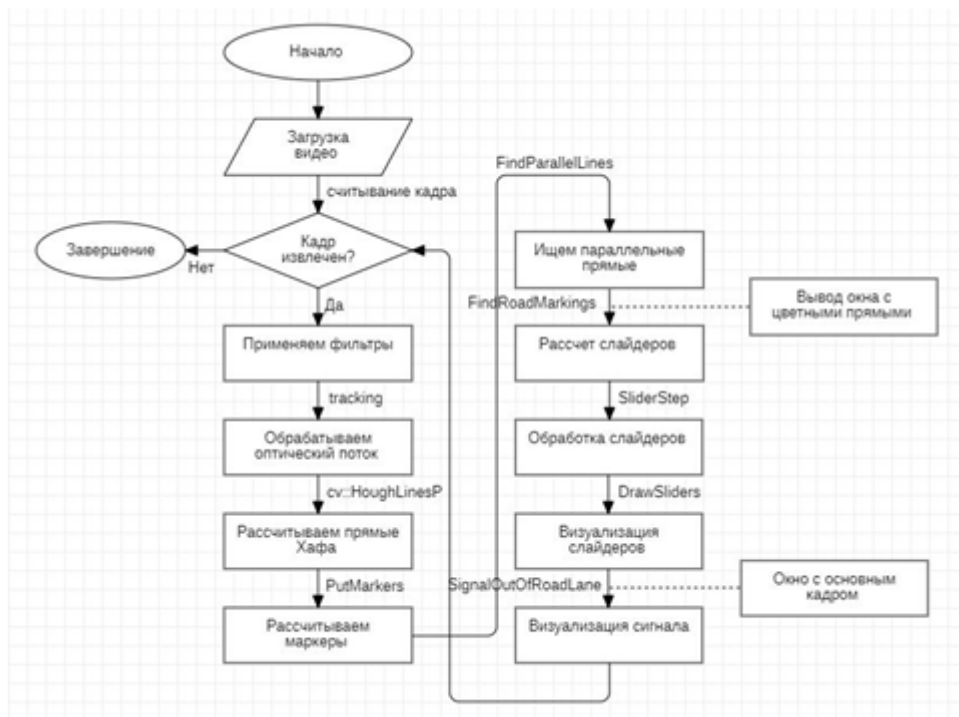
Рис. 1. Блок-схема
