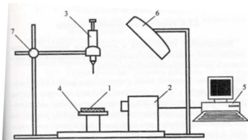
Рисунок 1.Схема установки для определения краевого угла смачивания
