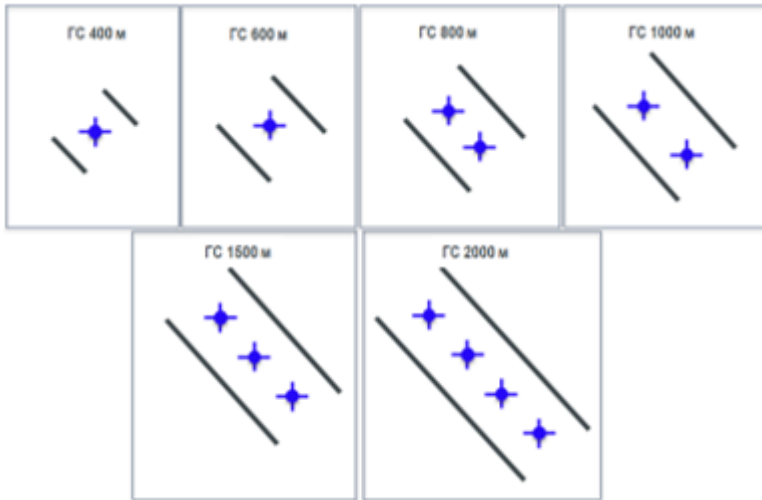
Рисунок 4. Элементы разработки рассмотренных систем разработки ГС с МГРП / ННС с ГРП.
