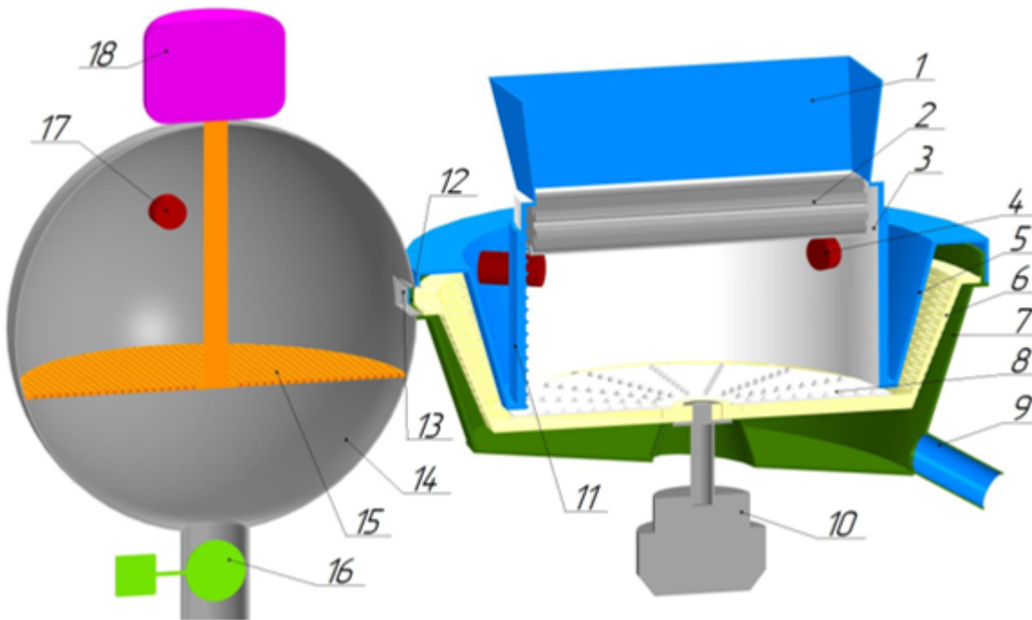
Рисунок 1 – СВЧ-установка для термообработки пчелиного воска:
