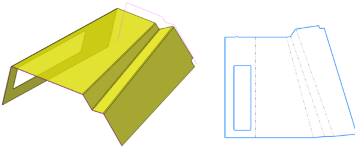
Рис.2 3D – модель и развертка элемента консоли
