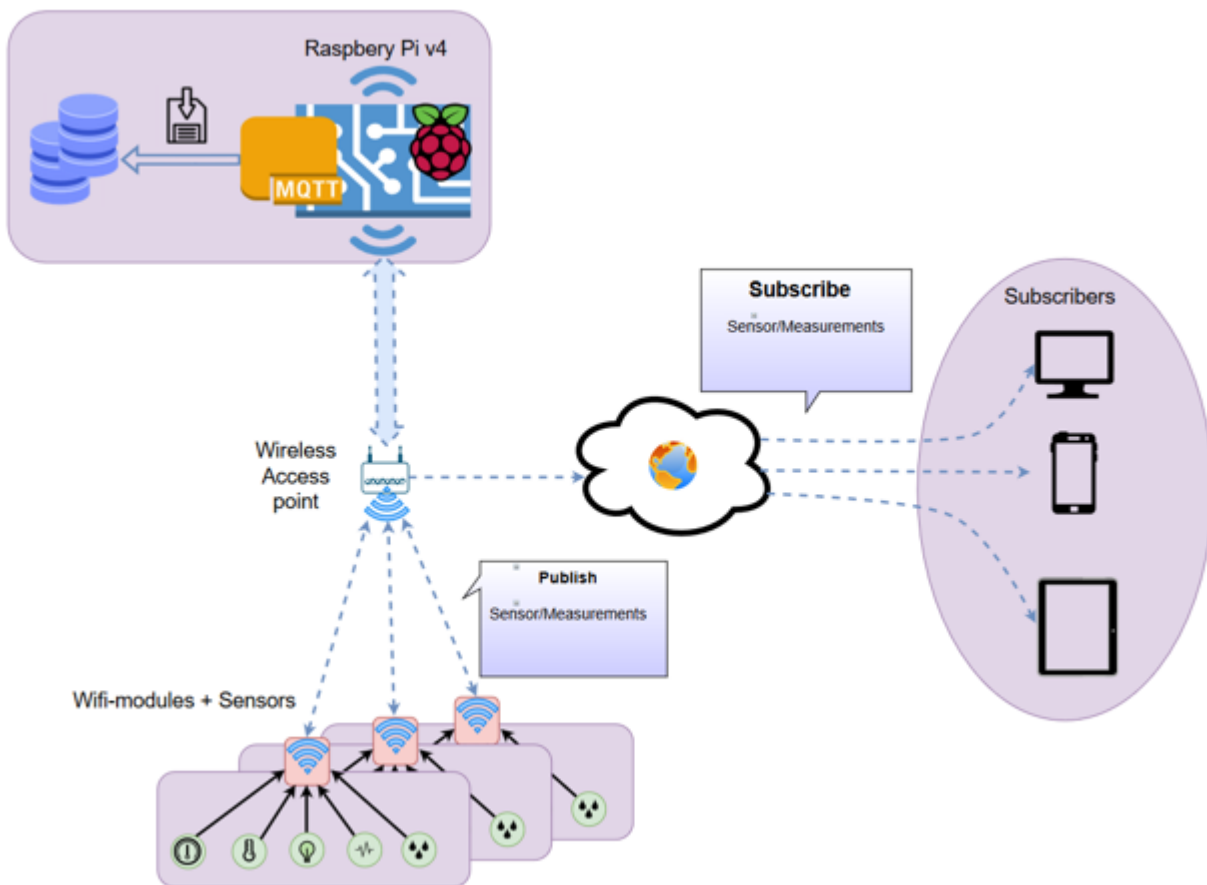
Рисунок 2. Модель системы датчиков мониторинга состояний помещений.
