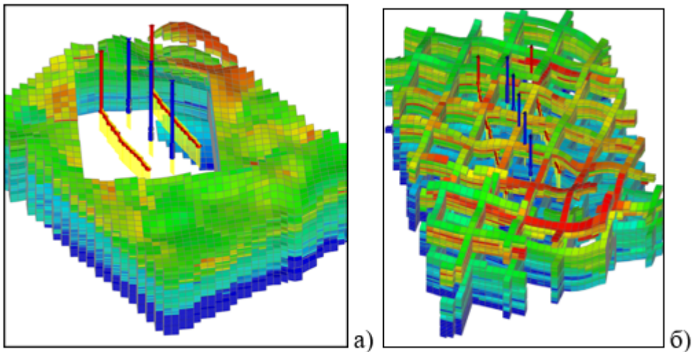
Рисунок 3. Разрезы куба нефтенасыщенности гидродинамической модели для элемента разработки с длиной ГС 1200 м (а) и 2000 м (б).
