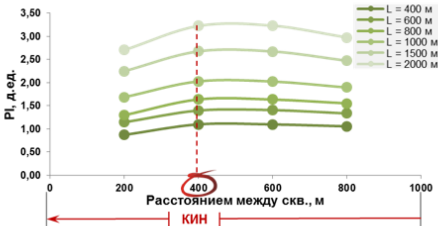
Рисунок 5. Индекс доходности инвестиций в зависимости от расстояния между рядами скважин для различных длин ГС.
