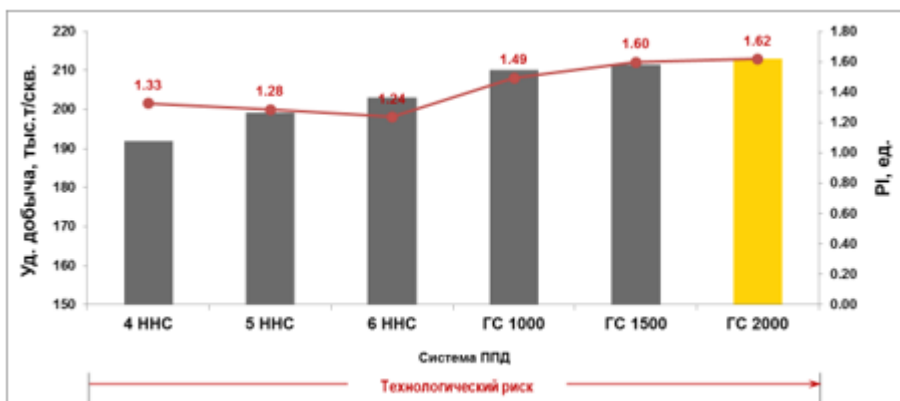
Рисунок 5. Диаграмма удельной накопленной добычи на скважину для элемента ГС длиной 2000м и индекса доходности инвестиций (PI) на элемент разработки, в зависимости от типа нагнетательной скважины/скважин.
