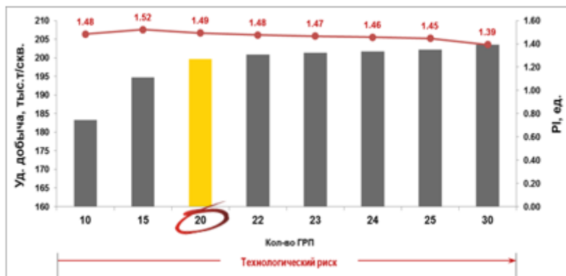
Рисунок 3. Диаграмма удельной накопленной добычи на скважину длиной 2000м и индекса доходности инвестиций (PI) на элемент разработки в зависимости от количества ГРП на скважине.
