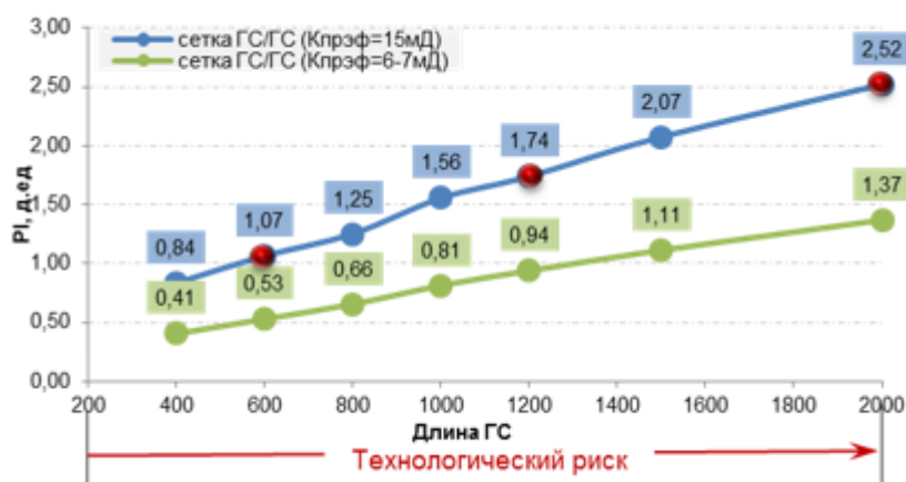
Рисунок 1. Индекс доходности инвестиций в зависимости от длины ГС для зон с эффективной проницаемостью 7 и 15 мД.
