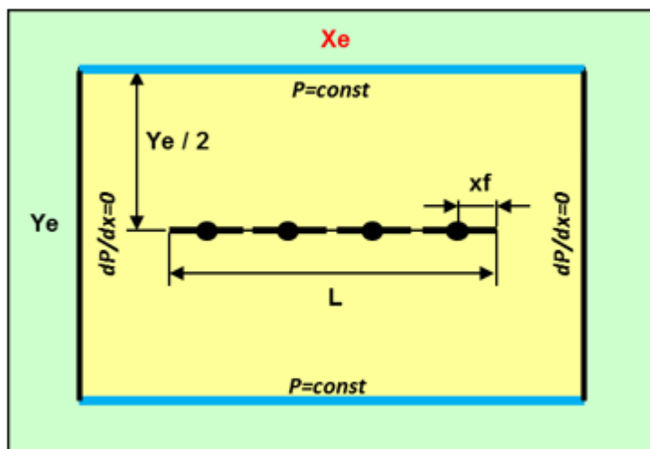
Рисунок 1. Схема расчета системы трещин ( X_e – расстояние между рядами скважин, Y_e – длина ГС + расстояние между скважинами в ряду, L – длина горизонтального ствола, x_f = 50 м – полудлина трещины ГРП).
