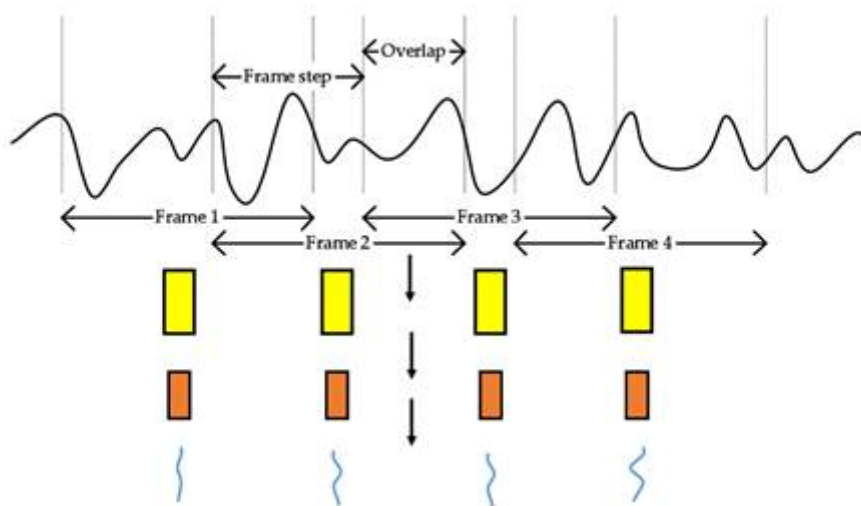
Рисунок 5. Предсказание фонем
