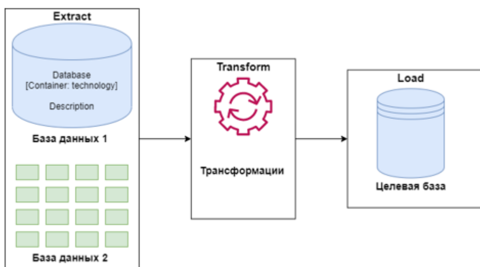
Рис. 1 ETL процесс
