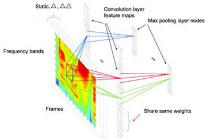
Рисунок. 7 Работа Сверточной нейронной сети
