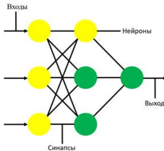
Рисунок 1. Нейронная сеть
