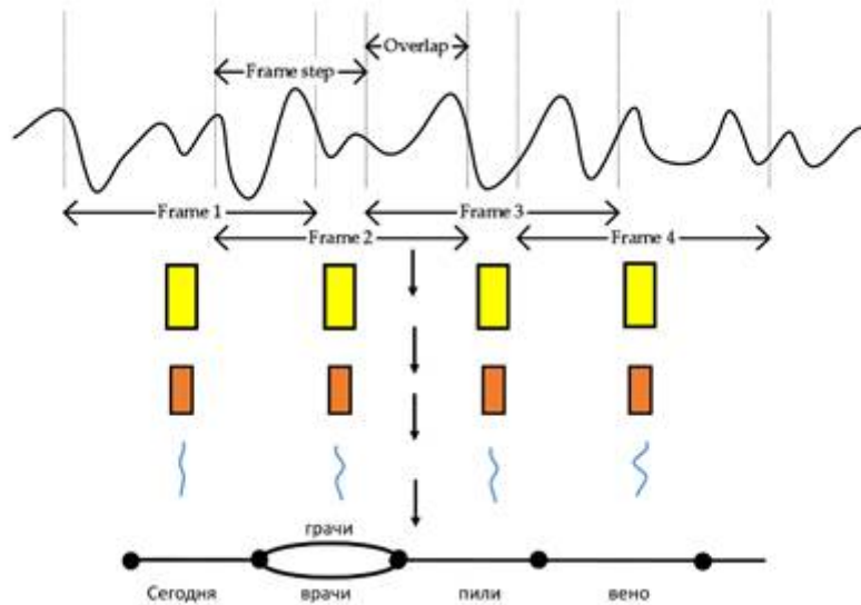
Рисунок. 6 Декодирование
