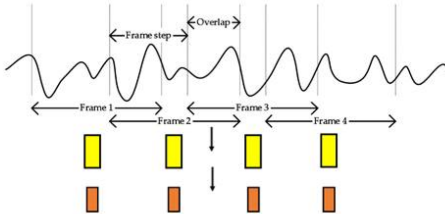
Рисунок 4. Выделения признаков
