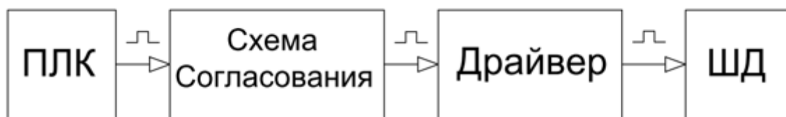
Рисунок 5 – Структурная схема системы позиционирования на основе ШД
