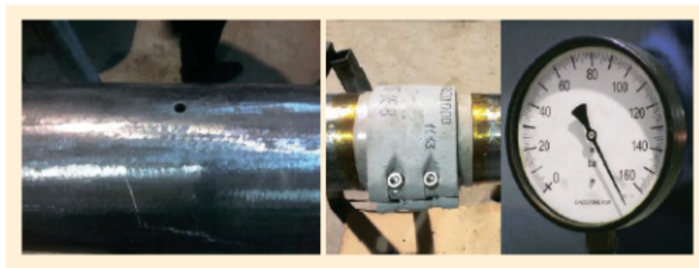
Рис.1. Аварийный ремонт сквозных отверстий с помощью УКМТ168
