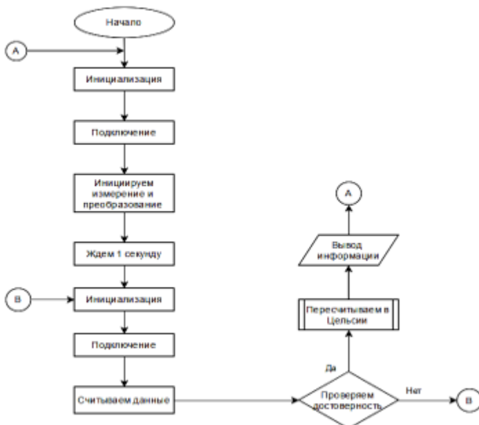
Рисунок 4. Блок-схема алгоритма кода DS18B20
