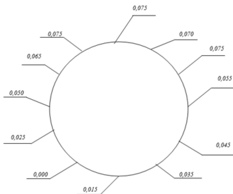
Рисунок 1 - Нивелирная съемка крайки днища
